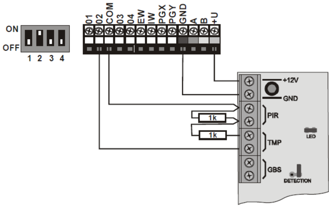
Fig. 2: Wiring a JS-20
