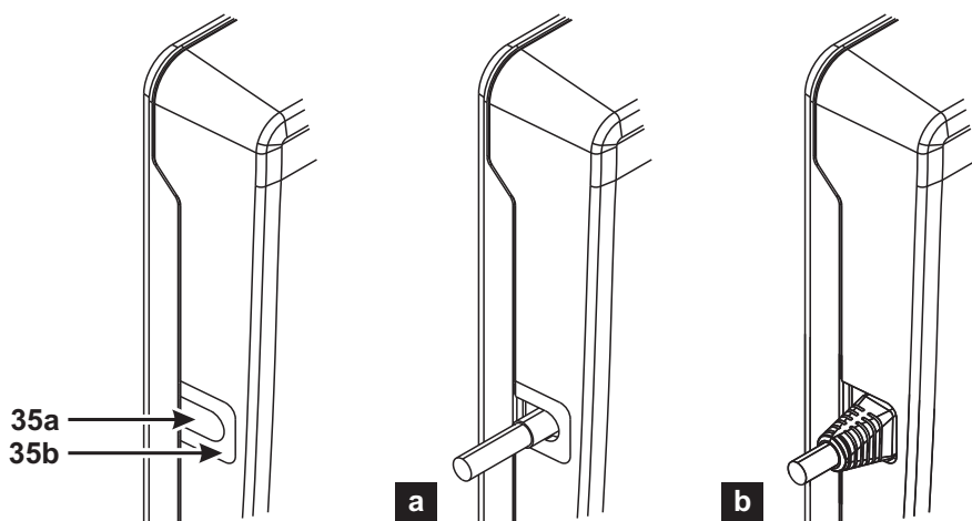
Figure 4 – Installation du transmetteur avec boîtier.
