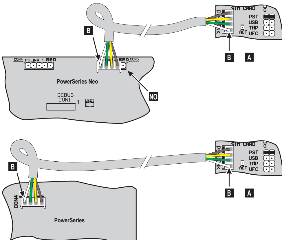
Figure 11 – Connexion du transmetteur à la centrale à l'aide du câble PCLINK-PCLINK : A) Transmetteur ; B) fil blanc.
