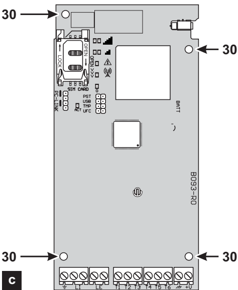
Figure 2 – Identification des pièces : a) version avec boîtier ; b) ANTLTE-02, antenne multibande avec câble de 2 m et connecteur SMA (en option) ; c) version en kit.
