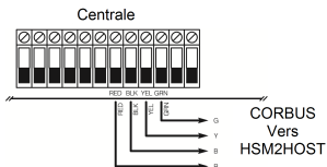
Figure : 1 Schéma de câblage
