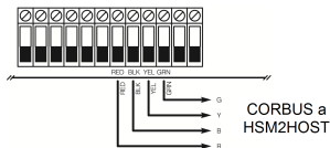
Figura: 1 Diagrama de cableado
