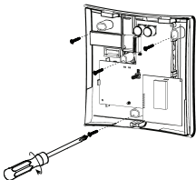
Figure : 1 Fixation du module HSM2HOST
