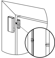
Figura 3: Posição do dispositivo e do ímã na porta e batente
