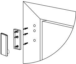
Figura 5: Dispositivo de instalación de tornillo
