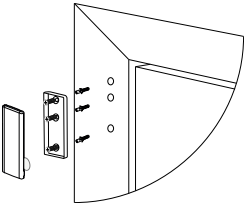
Figura 5: Instalação do parafuso do dispositivo
