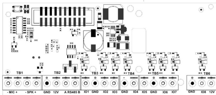
Schéma 2.2 - Emplacement des raccordements
